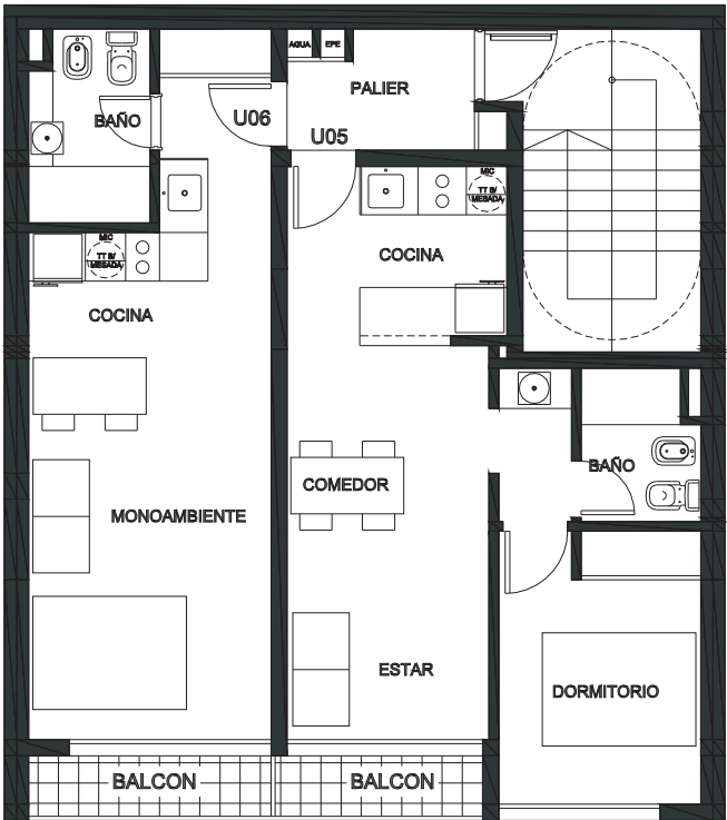
PLANTA TIPO PISOS 1 A 3
