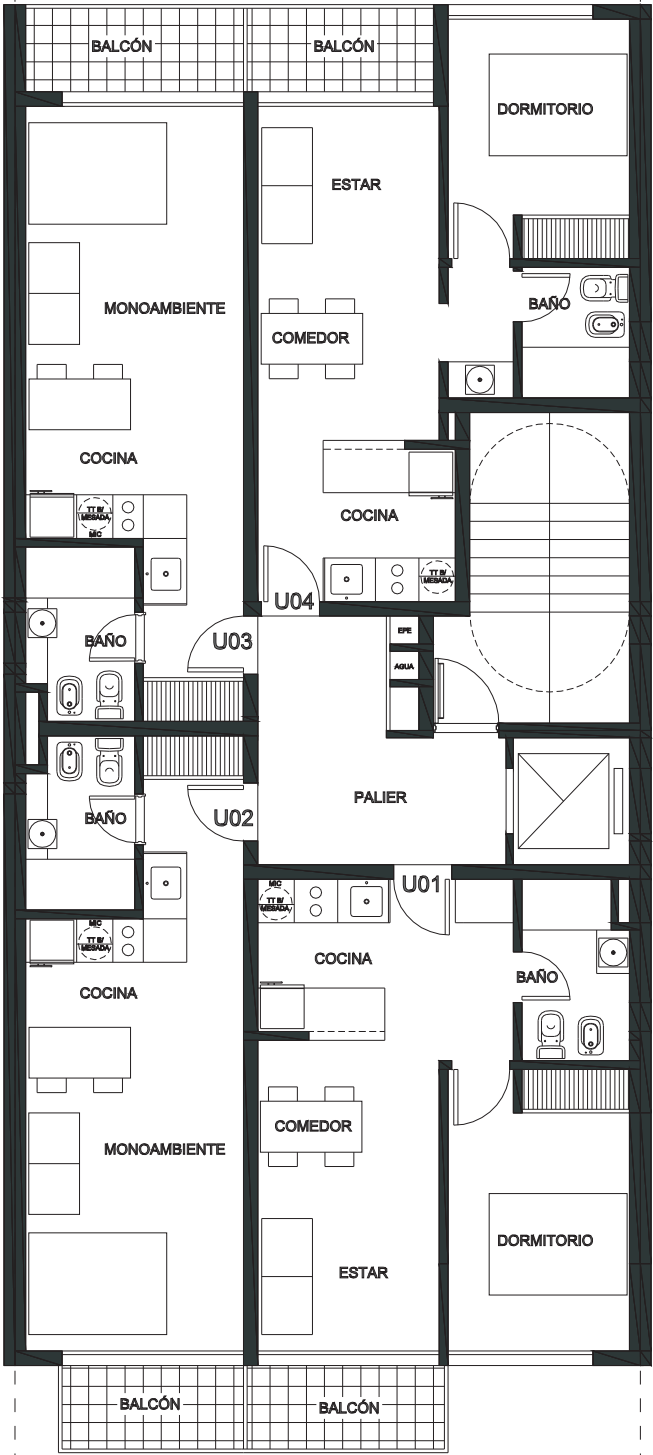
PLANTA TIPO PISOS 1 A 10
