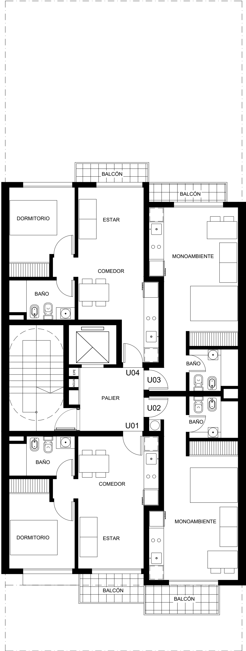
PLANTA TIPO 1 A 8 PISO
